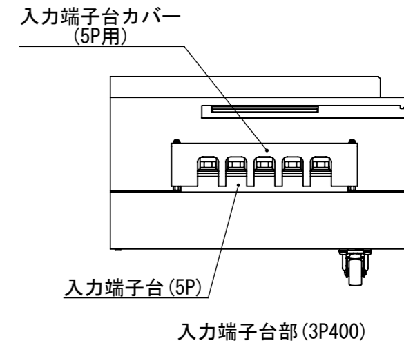
モデル別入力端子台部詳細
