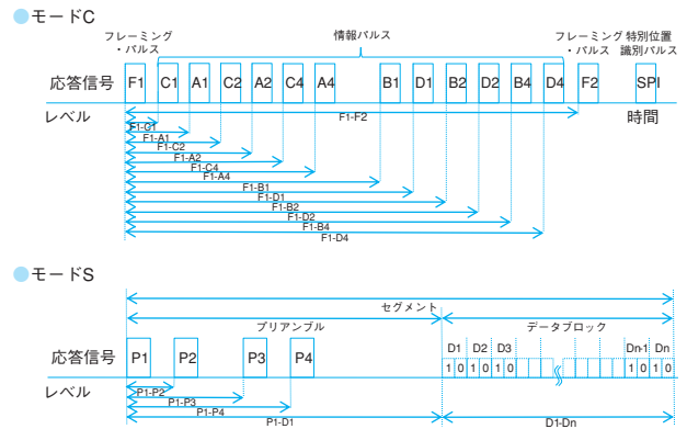
※図⑥ トランスポンダ 応答信号 パルス間隔
