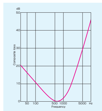
占有周波数帯幅測定用疑似音声フィルタの特性
